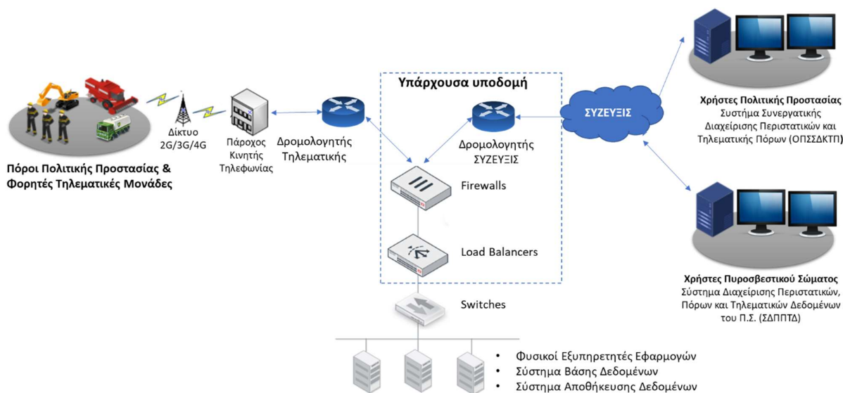
Εικόνα 1: Φυσική αρχιτεκτονική
